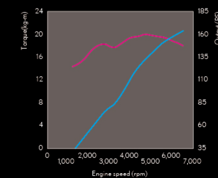
ES 200 引擎動力輸出曲線圖 6AR-FSE 2.0 升 L4 引擎
