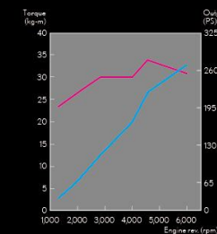
RX 450h 引擎動力輸出曲線圖 2GR-FXS 3.5 升 V6 Atkinson 循環引擎
