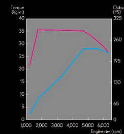
RX 200t 引擎動力輸出曲線圖
