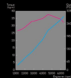
RX 350 引擎動力輸出曲線圖 2GR-FKS 3.5 升 V6 引擎
