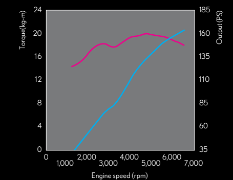
ES 200 引擎動力輸出曲線圖 6AR-FSE 2.0 升 L4 引擎
