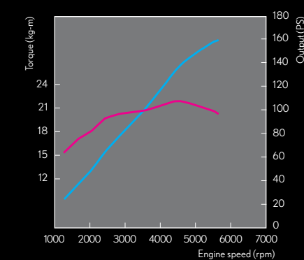
ES 300h 引擎動力輸出曲線圖 2AR-FXE 2.5 升 Atkinson 循環引擎
