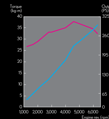
RX 350、RX 350L 引擎動力輸出曲線圖
