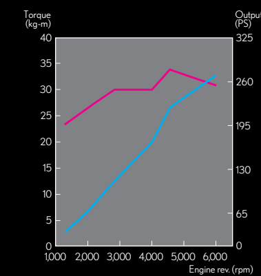
RX 450h、RX 450hL 引擎動力輸出曲線圖 2GR-FXS 3.5 升 V6 Atkinson 循環引擎
