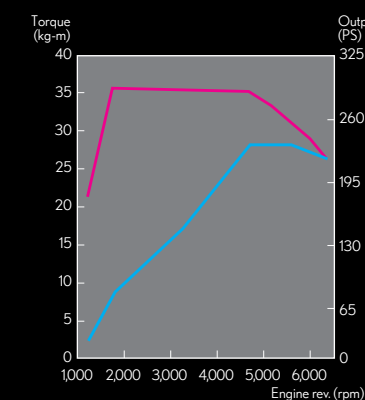
RX 300 引擎動力輸出曲線圖
