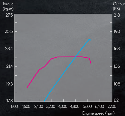
ES 300h 引擎動力輸出曲線圖
