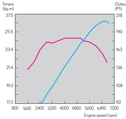
ES 250 引擎動力輸出曲線圖
