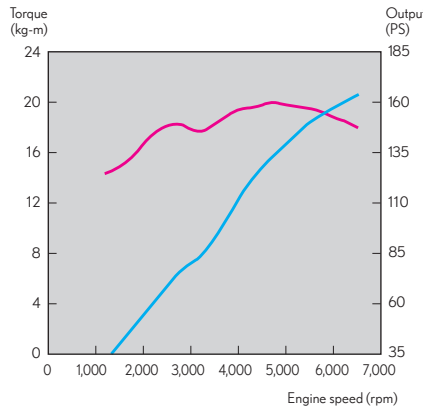
ES 200 引擎動力輸出曲線圖
