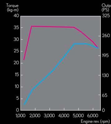
RX 300 引擎動力輸出曲線圖
