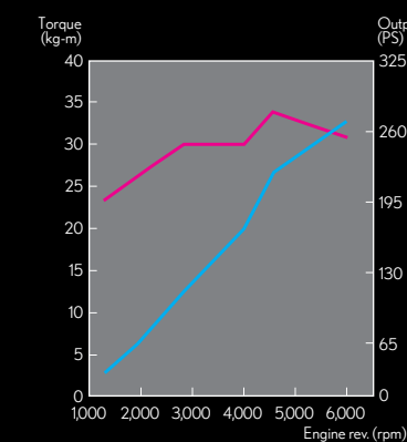
RX 450h、RX 450hL 引擎動力輸出曲線圖 2GR-FXS 3.5 升 V6 Atkinson 循環引擎
