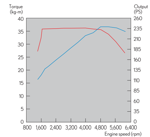
NX 300 引擎動力輸出曲線圖
