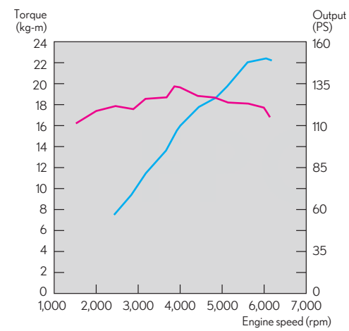
NX 200 引擎動力輸出曲線圖
