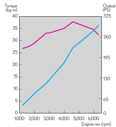
RX 350、RX 350L 引擎動力輸出曲線圖
