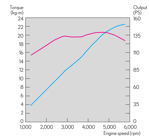
NX 300h 引擎動力輸出曲線圖
