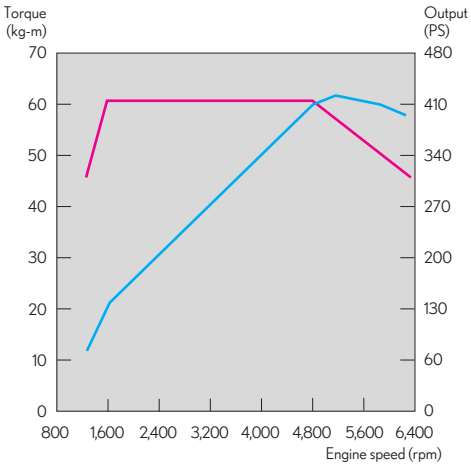
LS 500 引擎動力輸出曲線圖
