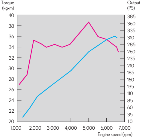
LS 350 引擎動力輸出曲線圖
