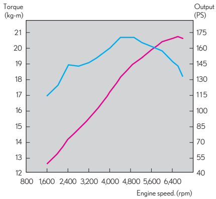
ES 200 引擎動力輸出曲線圖
