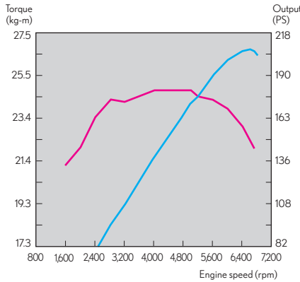
ES 250 引擎動力輸出曲線圖
