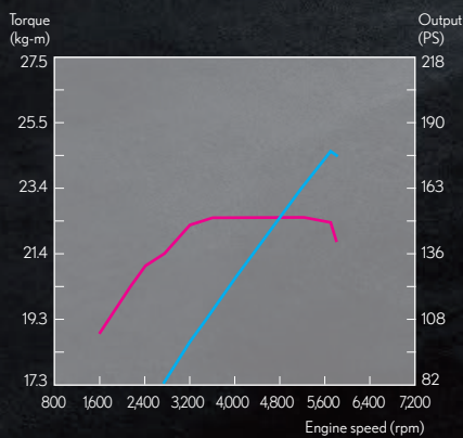
ES 300h 引擎動力輸出曲線圖
