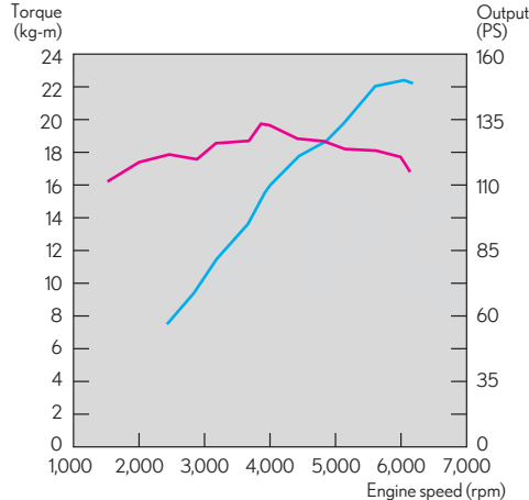
NX 200 引擎動力輸出曲線圖
