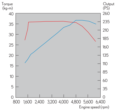
NX 300 引擎動力輸出曲線圖
