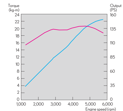
NX 300h 引擎動力輸出曲線圖
