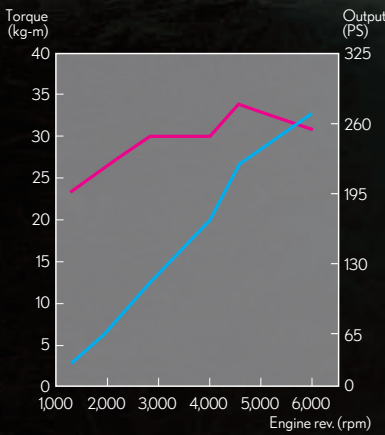
RX 450h、RX 450hL 引擎動力輸出曲線圖
