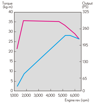
RX 300 引擎動力輸出曲線圖
